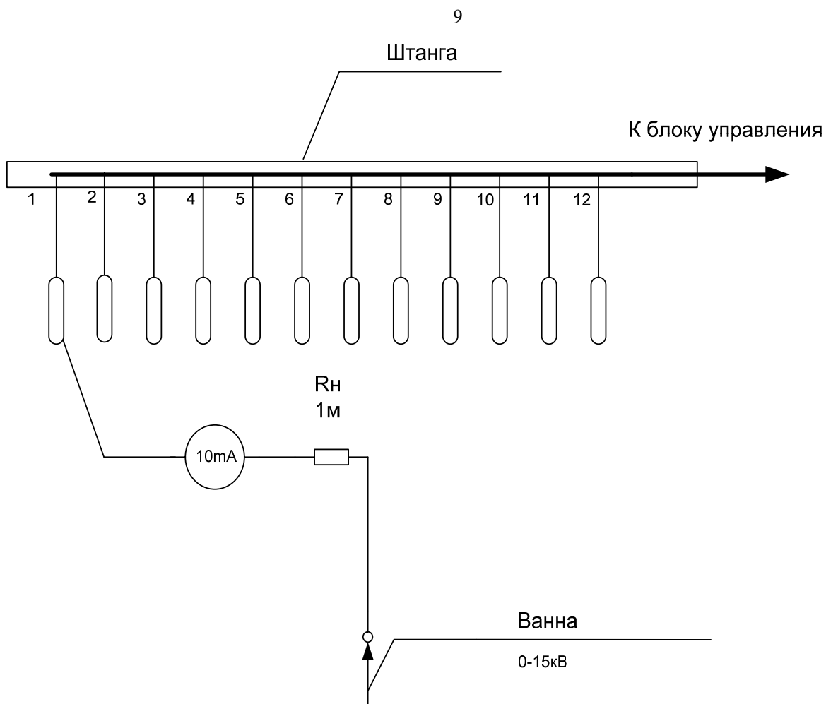
Рис.2 Схема подключений при калибровке тока защиты станда для каждой перчатки.
